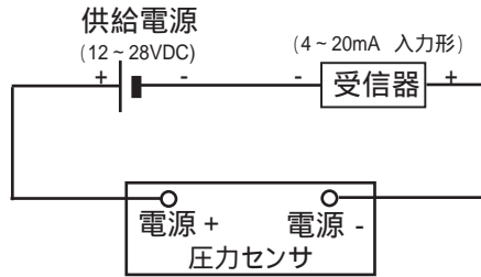
(配線参考図)
