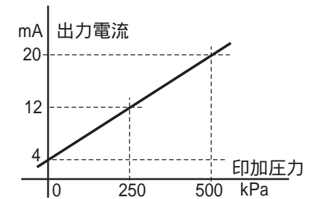
圧力-出力特性
